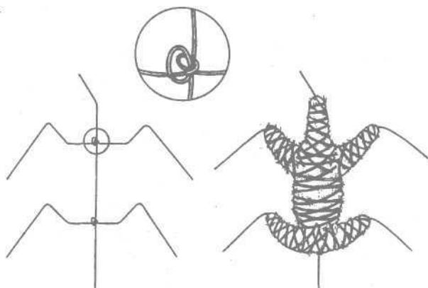
Проволочная основа, обмотанная тканью
